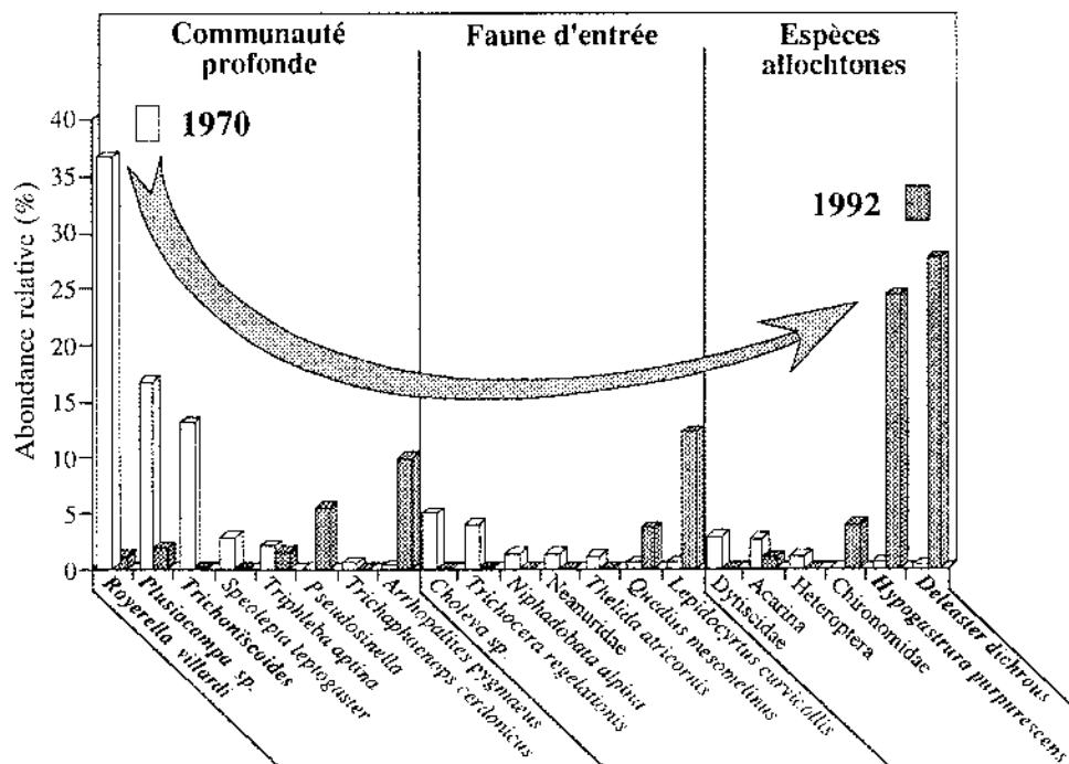
FIG. 3. - Évolution de l'abondance relative des principaux taxons terrestres au Puits de Rappe entre 1970 et 1992 (Turquin & Craguc, 1994).
